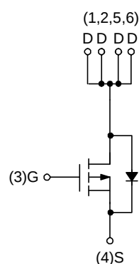
P-Channel MOSFET
