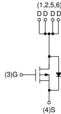
P-Channel MOSFET
