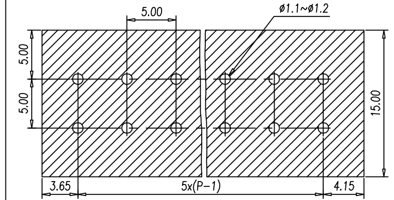
P.C.B. LAYOUT(REF)
