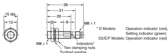
Diagram 28 E2E-X2D□-M3G/E2E-X1R5E□-M3/X1RF□-M3
