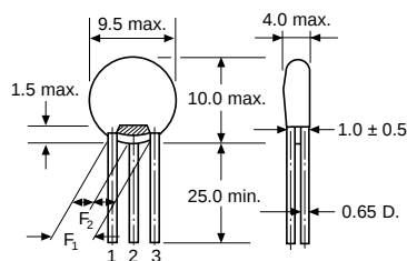
DS310/310H TYPE Fig. 1
