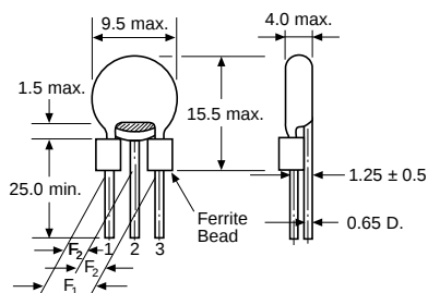
DST310/310H TYPE Fig. 2
