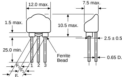
DSS310/310H TYPE Fig. 3
