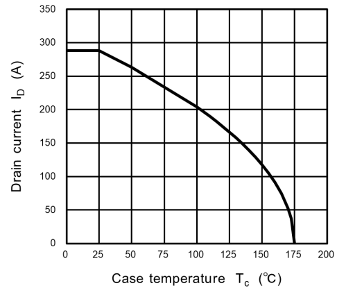
Fig. 8.15 I_D - T_c
