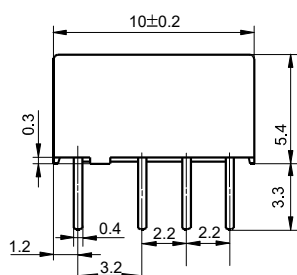
THT type
