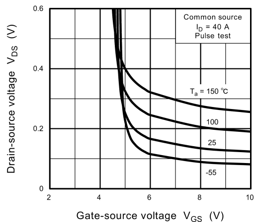
Fig. 8.3 V_{DS} - V_{GS}
