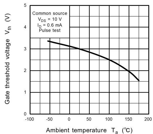
Fig. 8.12 V_{th} - T_a
