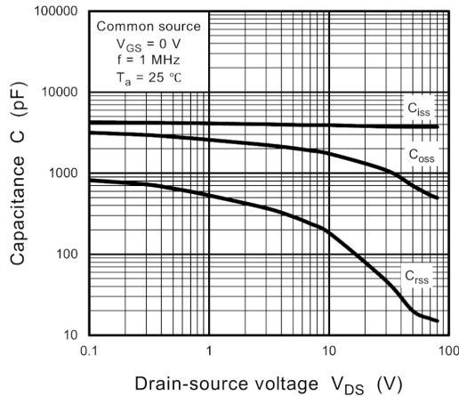
Fig. 8.13 Capacitance - V_{DS}
