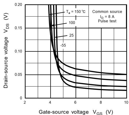
Fig. 8.5 V_{DS} - V_{GS}
