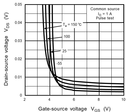
Fig. 8.6 V_{DS} - V_{GS}
