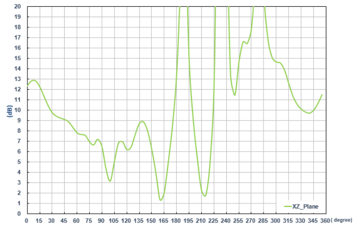
@1602MHz
