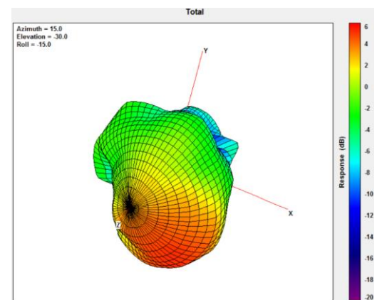
2690MHz
