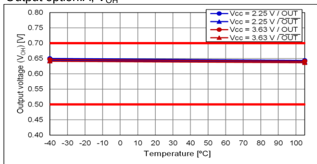
Output option:A, V_{OH}
