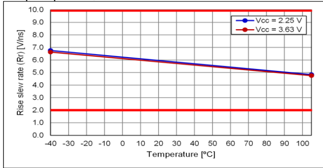
Output option:A, Rise Slew Rate
