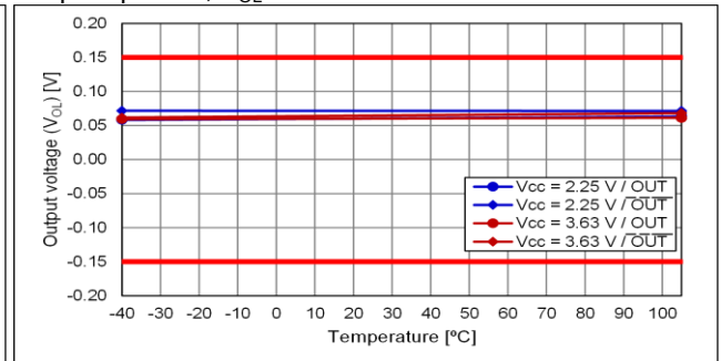
Output option:B, V_{OL}
