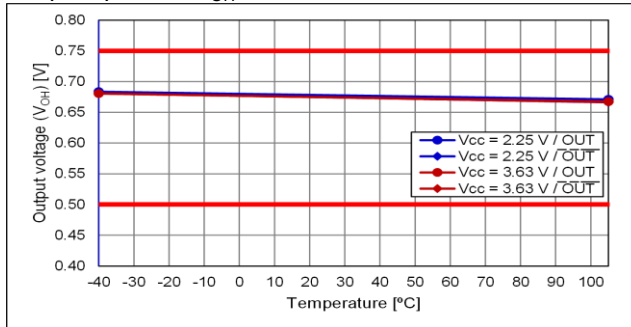
Output option:B, V_{OH}
