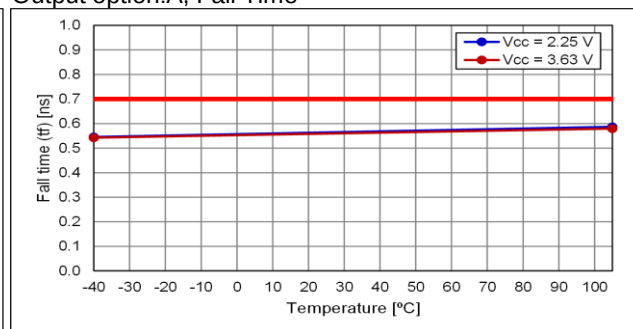
Output option:A, Fall Time
