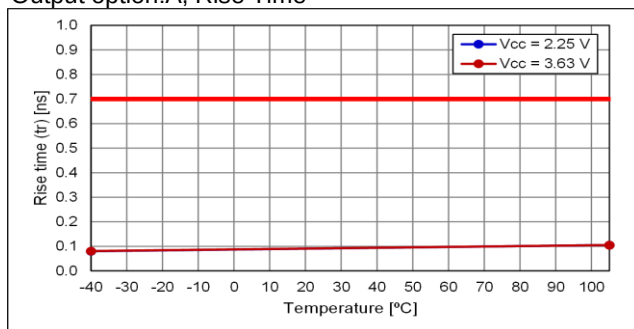
Output option:A, Rise Time
