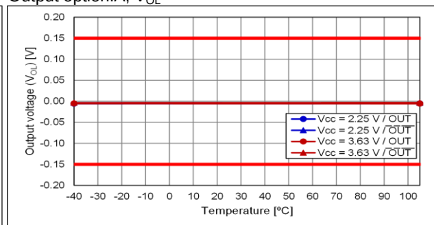
Output option:A, V_{OL}
