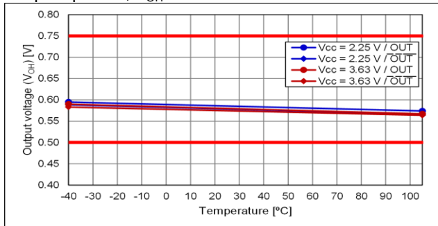
Output option:B, V_{OH}
