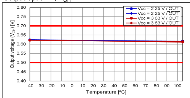
Output option:A, V_{OH}
