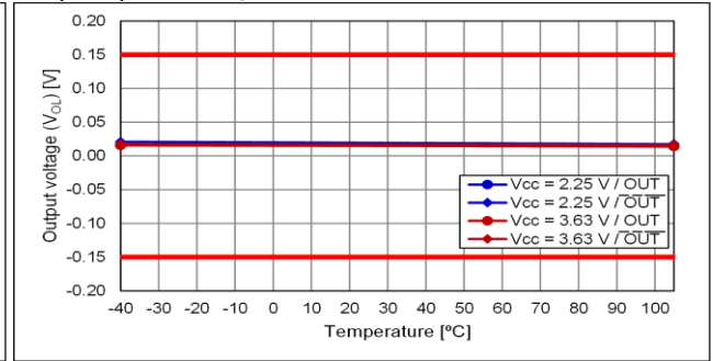
Output option:A, V_{OL}
