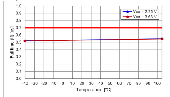
Output option:A, Fall Time
