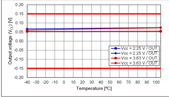
Output option:A, V OL
