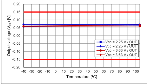
Output option:B, V OL
