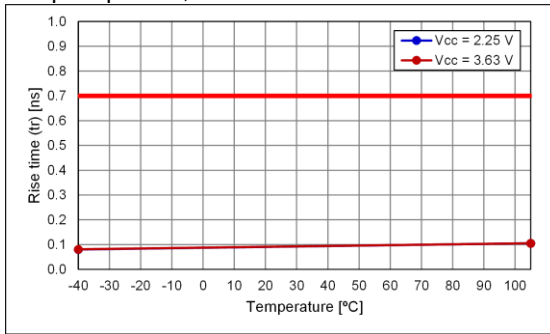
Output option:B, Rise Time
