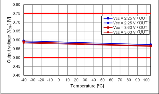
Output option:B, V OH
