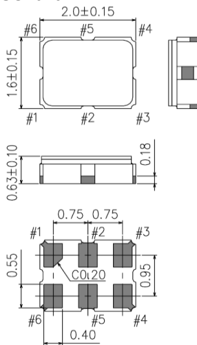
SG2016EHN
