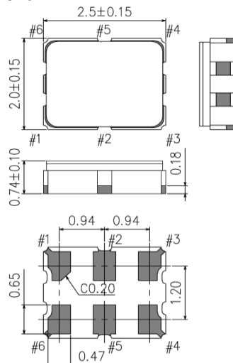
SG2520EHN
