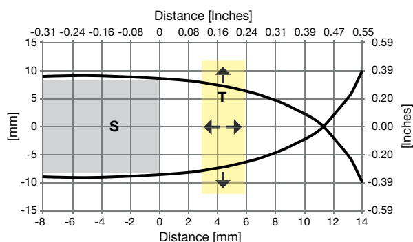
Fig. 4 M18 Non-flush
