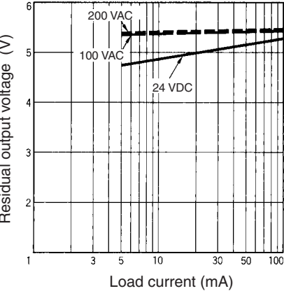
E2E-X□T1
