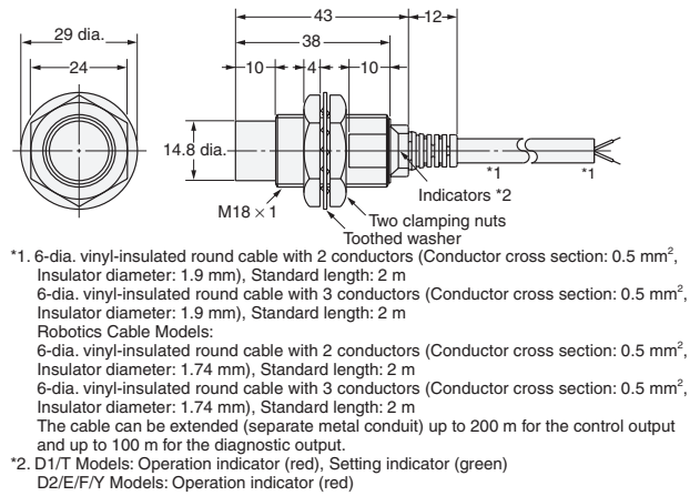
Diagram 11 E2E-X14MD□/E2E-X10ME□/F□ E2E-X10MY□
