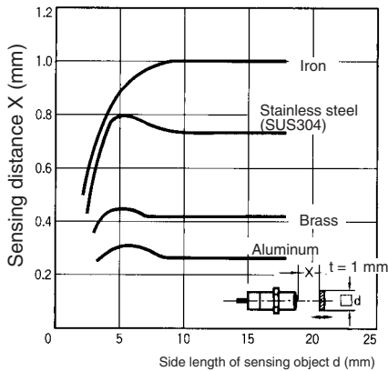
E2E-X1□□ E2E-C1□□
