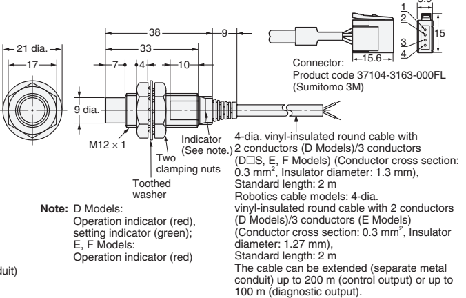
Fig. 10: E2E-X8MD□ E2E-X5ME□/F□
