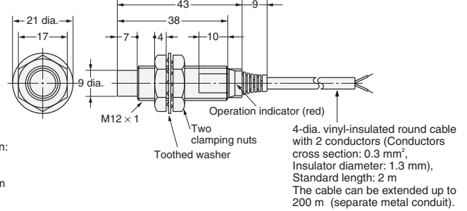
Fig. 12: E2E-X5MY□
