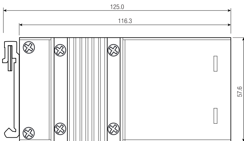
DIN Rail Version (mm)
