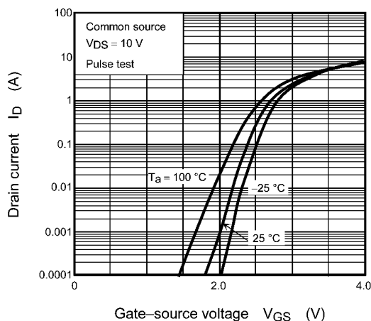
Fig. 9.2 I_D - V_{GS}
