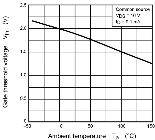
Fig. 9.7 V_{th} - T_a
