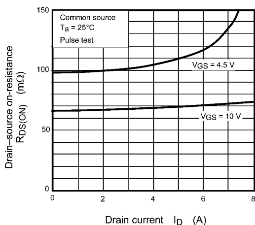
Fig. 9.5 R_{DS(ON)} - I_D
