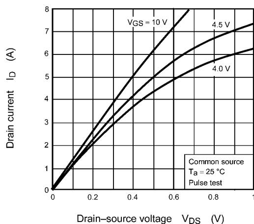
Fig. 9.1 I_D - V_{DS}
