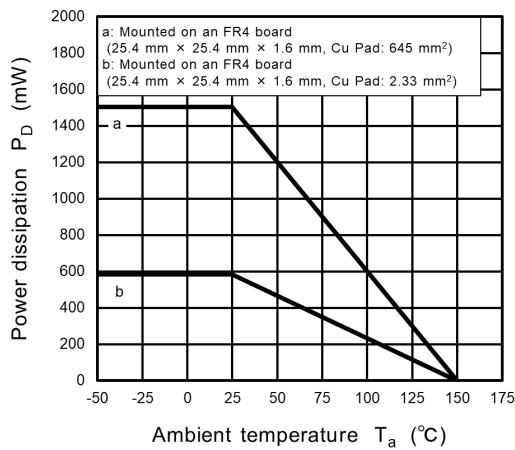
Fig. 9.10 P_D - T_a
