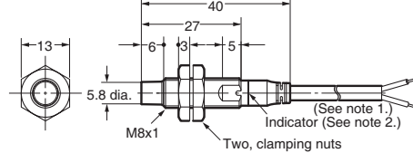
E2A-S08KN04-WP-□□
