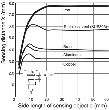
E2A-S18□S08
