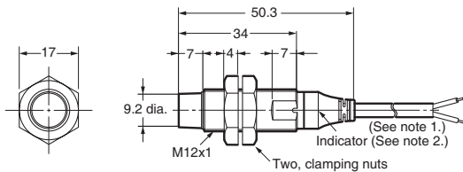
E2A-S12KN08-WP-□
