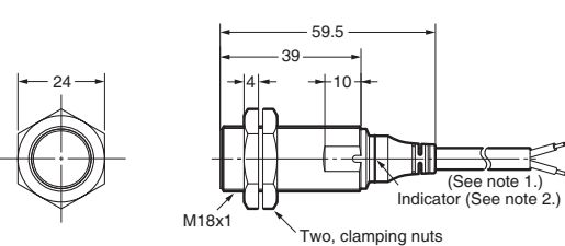
E2A-S18KS08-WP-□
