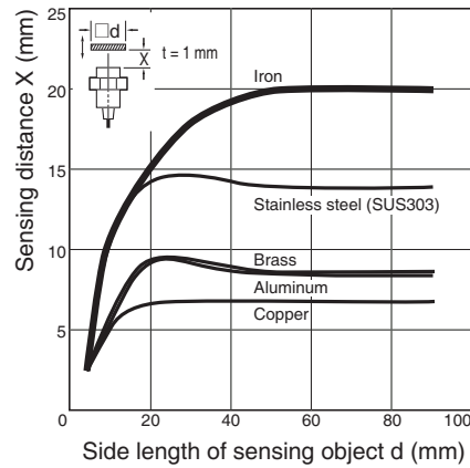
E2A-S30KN20
