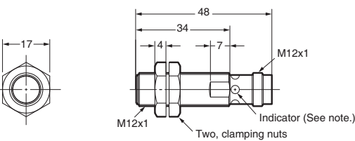
E2A-S12KS04-M1-□
