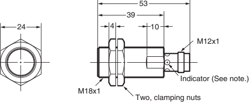
E2A-S18KS08-M1-□
