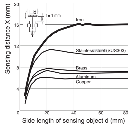
E2A-S18□N16
