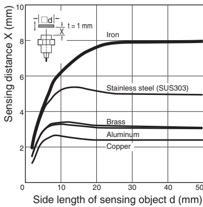
E2A-S12□N08
