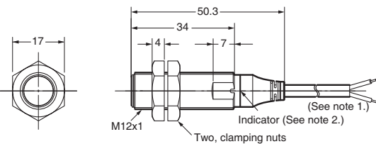
E2A-S12KS04-WP-□
