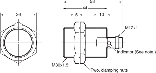
E2A-S30KS15-M1-□
