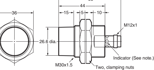
E2A-S30KN20-M1-□
