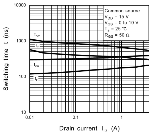
Fig. 9.9 t - I_D
