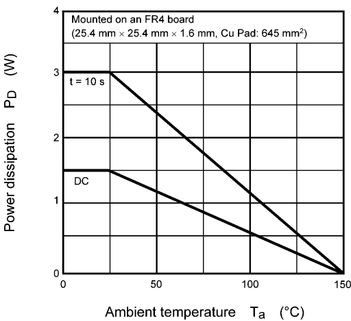
Fig. 9.12 P_D - T_a
