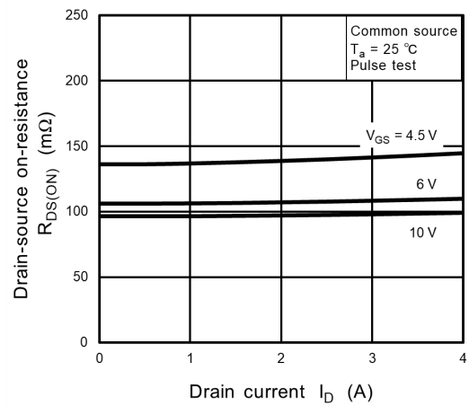
Fig. 9.4 R_{DS(ON)} - I_D
