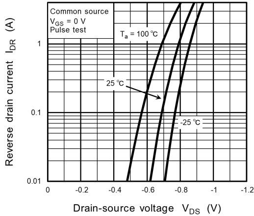
Fig. 9.7 I_{DR} - V_{DS}
