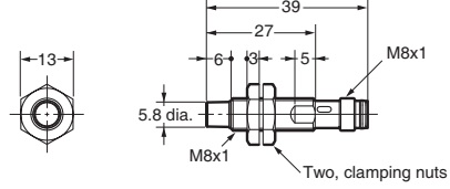
E2A-S08KN04-M5-□□/ E2A-S08KN04-M3-□
