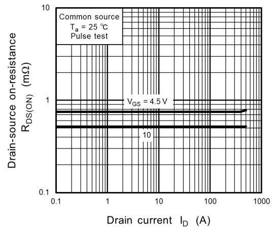
Fig. 8.4 R_{DS(ON)} - I_D
