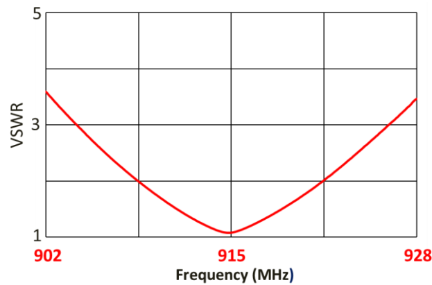
VSWR
