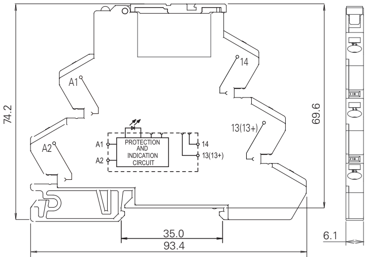
RV8S-S Spring Clamp Terminal (mm)
