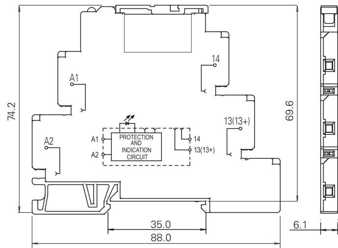
RV8S-L Screw Terminal (mm)
