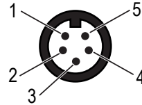
5-pin Mini male pinout
