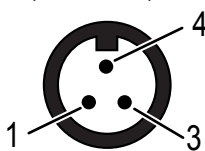
3-pin Mini male pinout
