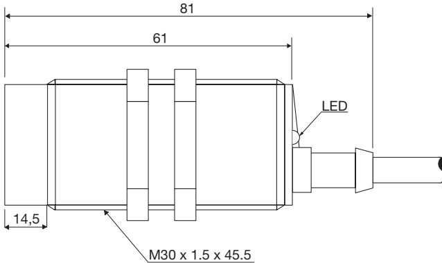
Fig. 7 Cable CA30CAN...A2IO
