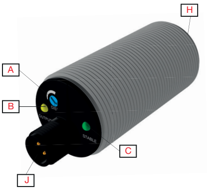
Fig. 2 CA30 Plug
