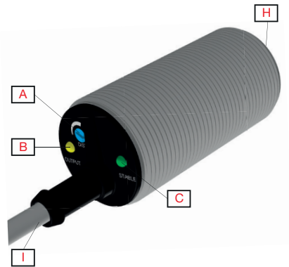
Fig. 1 CA30 Cable
