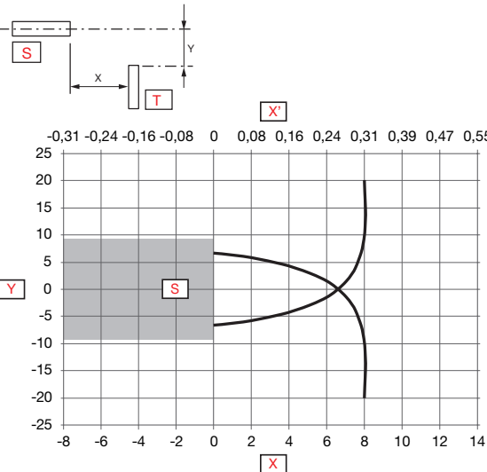
Fig. 4 Flush
