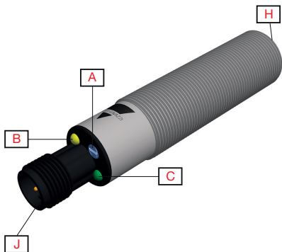
Fig. 2 CA18 Plug
