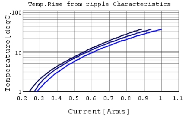
GJM1555C1H5R6DB01 Temp.rise 1GHz 2
