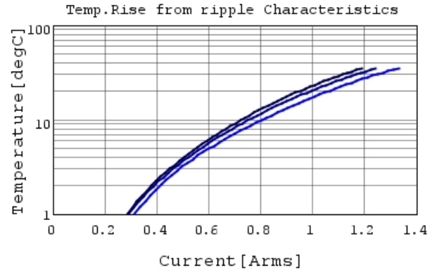
GQM1875C2E390JB12 Temp.rise 500MHz
