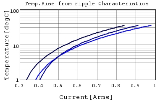
GJM0335C1E4R7WB01 Temp.rise — 2GHz — 3
