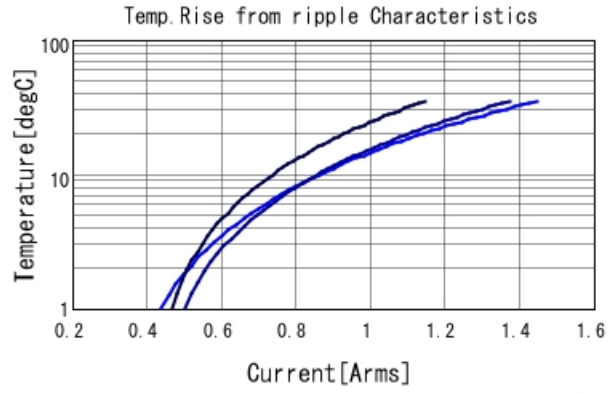
GQM1875G2E9R1BB12 Temp. rise ■ 700MHz ■ 1GHz ■ 2GHz
