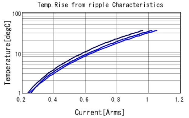
GQM1875G2E3R3WB12 Temp. rise — 1GHz — 2GHz
