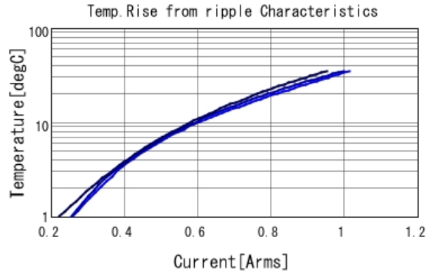
GQM1875G2E2R7BB12 Temp. rise — 1GHz — 2GHz
