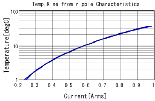
GQM1875G2E1R8BB12 Temp. rise ■ 2GHz ■ 3GHz
