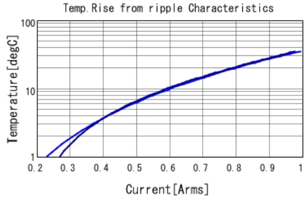
GQM1875G2E1R6WB12 Temp. rise — 2GHz — 3GHz
