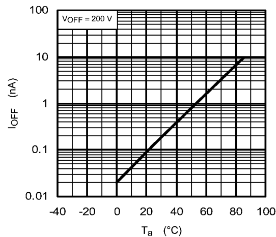
Fig. 16.9 I_{OFF} - T_a
