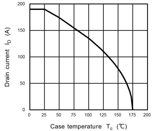
Fig. 8.15 I_D - T_c
