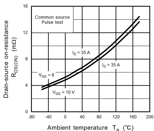
Fig. 8.9 R_{DS(ON)} - T_a
