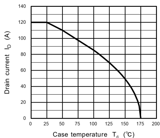
Fig. 8.15 I_D - T_c
