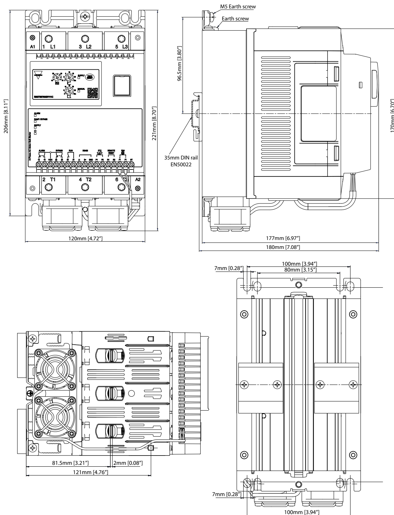
Fig. 3 RSGT 120mm: RSGT..70.. to RSGT..90
