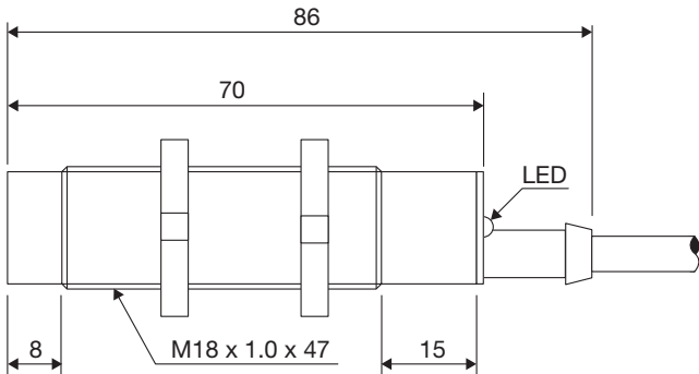
Fig. 7 Cable CA18EAN...A2IO
