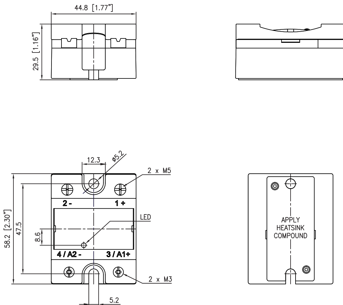
Fig. 1 RM1D dimensions
