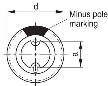
KAL1934-H-E
