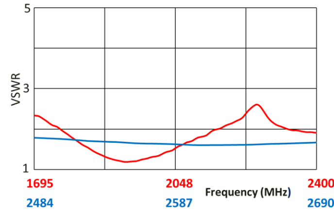
VSWR
