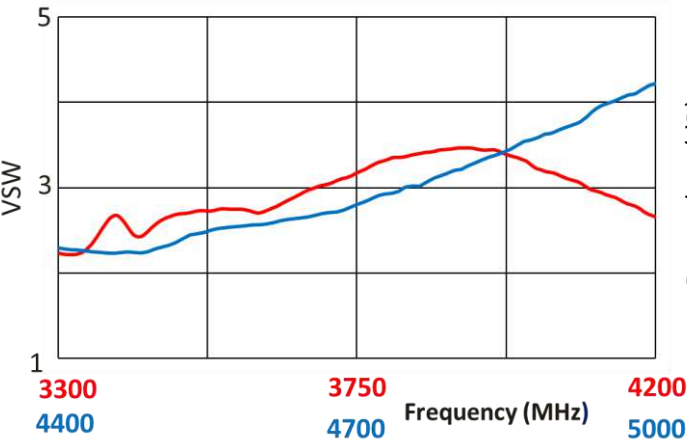
VSWR
