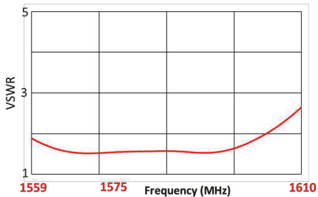
VSWR
