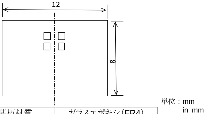
第5図 たわみ試験用基板 Figure 5. Test Board for Bending Strength Test
