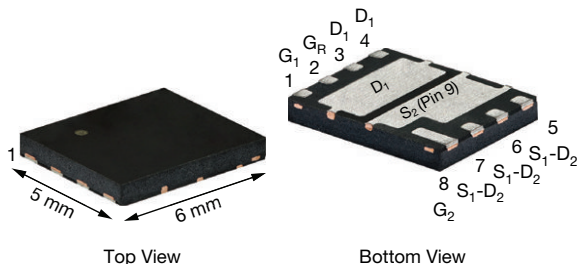
PowerPAIR® 6 x 5FSW
