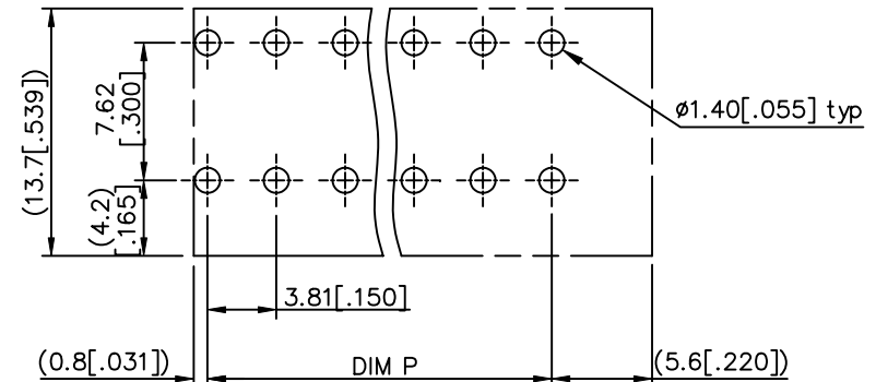
P.C.B. LAYOUT
