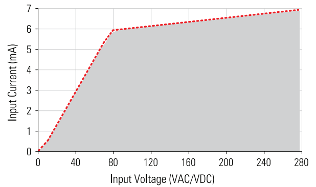
90-280 VAC/VDC Input
